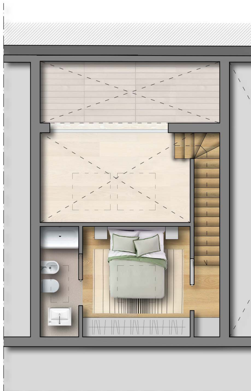
PIANTA PRIMO LIVELLO
